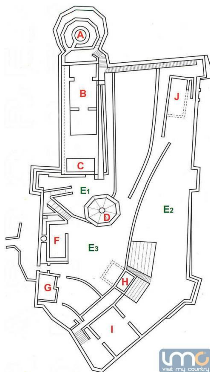
Slika 2: Tlocrt tvrđave Stari grad u Travniku
